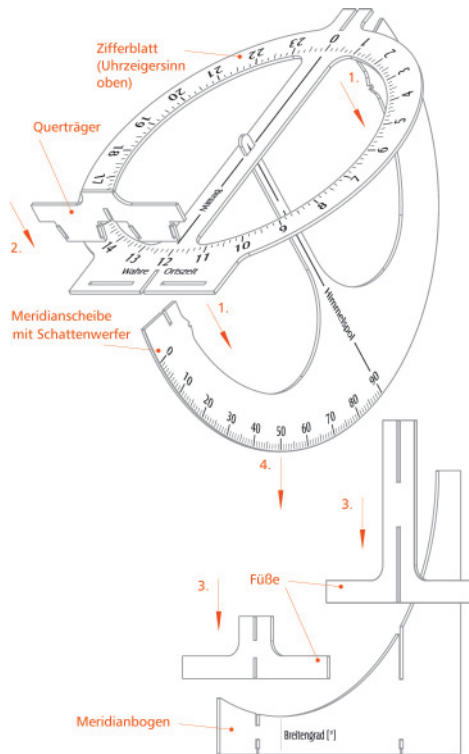
Bild 1: Zusammenbau in vier Schritten
